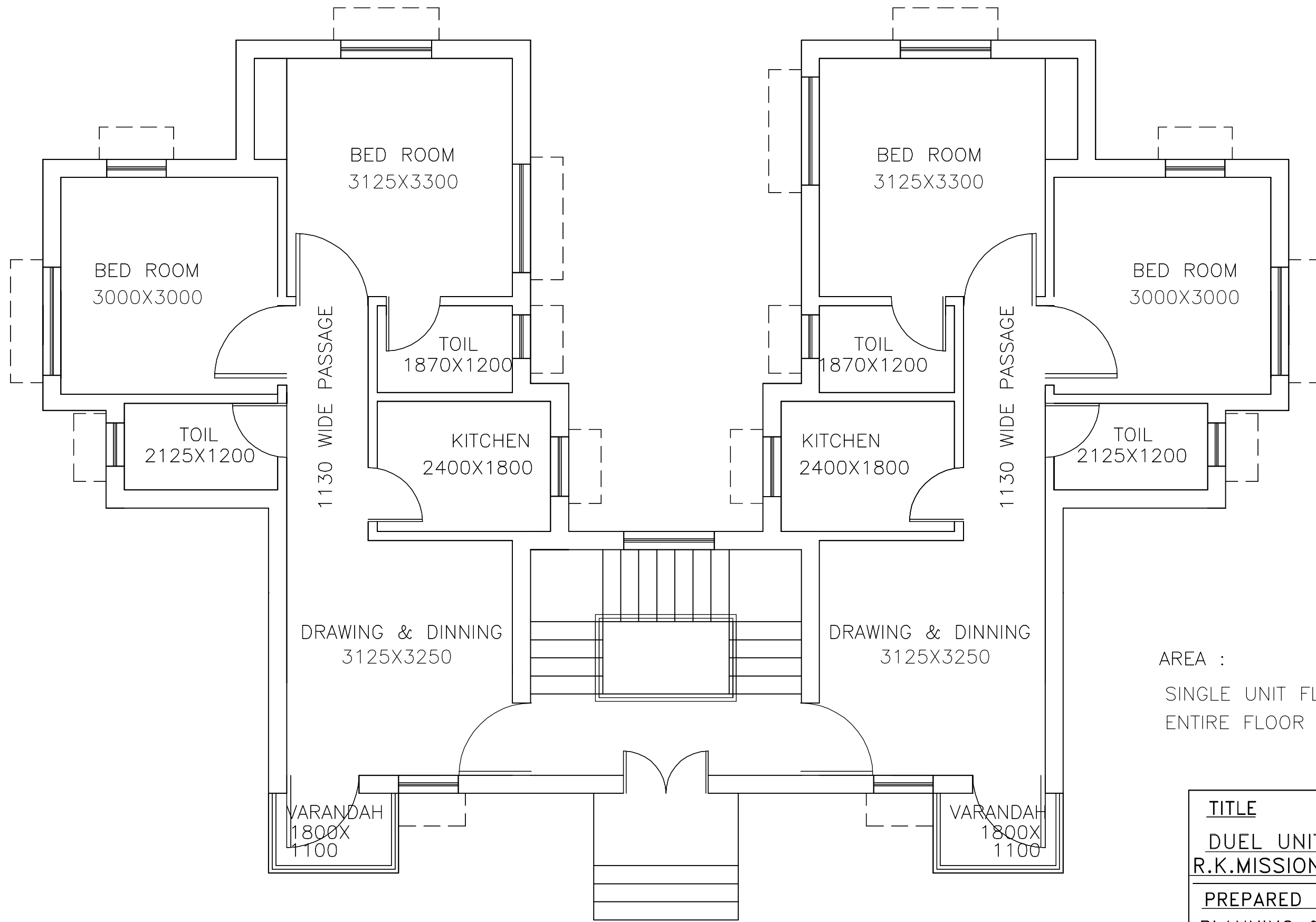
DUEL UNIT PLAN
